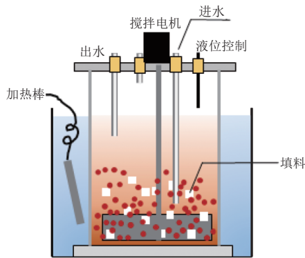
图 1 SBBR 示意图
