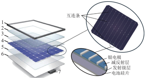
注: 1—铝边框; 2—玻璃; 3—上层 EVA; 4—太阳能电池; 5—下层 EVA; 6—背板; 7—接线盒。
