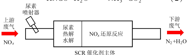
图1 尿素SCR技术工作原理
