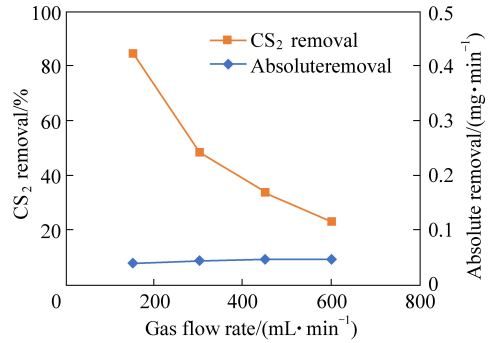
(b) 不同气体流量下的CS 2 去除效果
