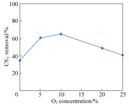
图 5 氧气浓度对二硫化碳去除效果的影响
