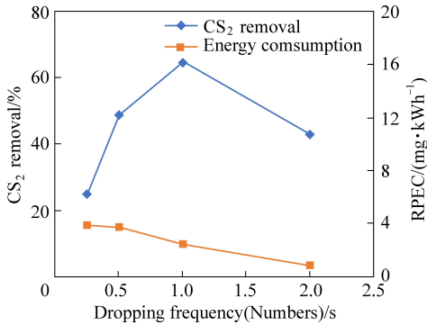
图 4 液滴滴加频率对二硫化碳去除效果和能耗的影响
