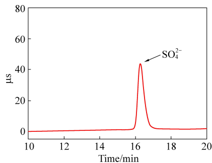
图8 CS 2 降解反应后的液相产物的离子色谱
