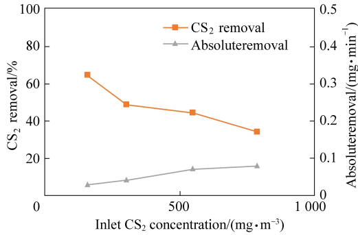
(a) 不同CS 2 初始浓度的去除效果
