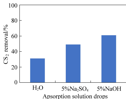
图6 液滴组分对二硫化碳去除效果的影响 (CS 2 初始浓度为300 mg/m 3 , 氧气浓度为20%)
