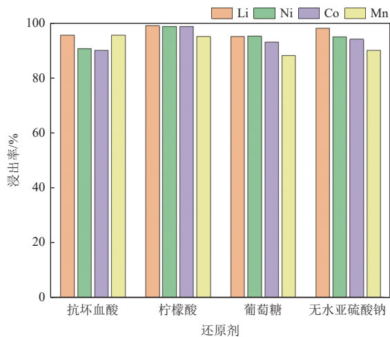
图 4 不同还原剂作用下不同金属的浸出率 [33]
