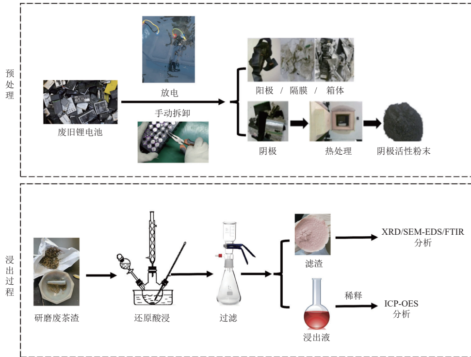
图 6 茶渣浸出废旧锂电池中有价金属实验过程 [44]
