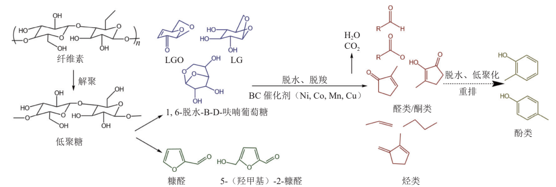
图 3 纤维素生成还原性气体的机理 [19]
