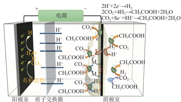
图2 MES转化CO 2 为乙酸的工作原理图 Fig. 2 Schematic diagram of MES for converting CO 2 to acetate
