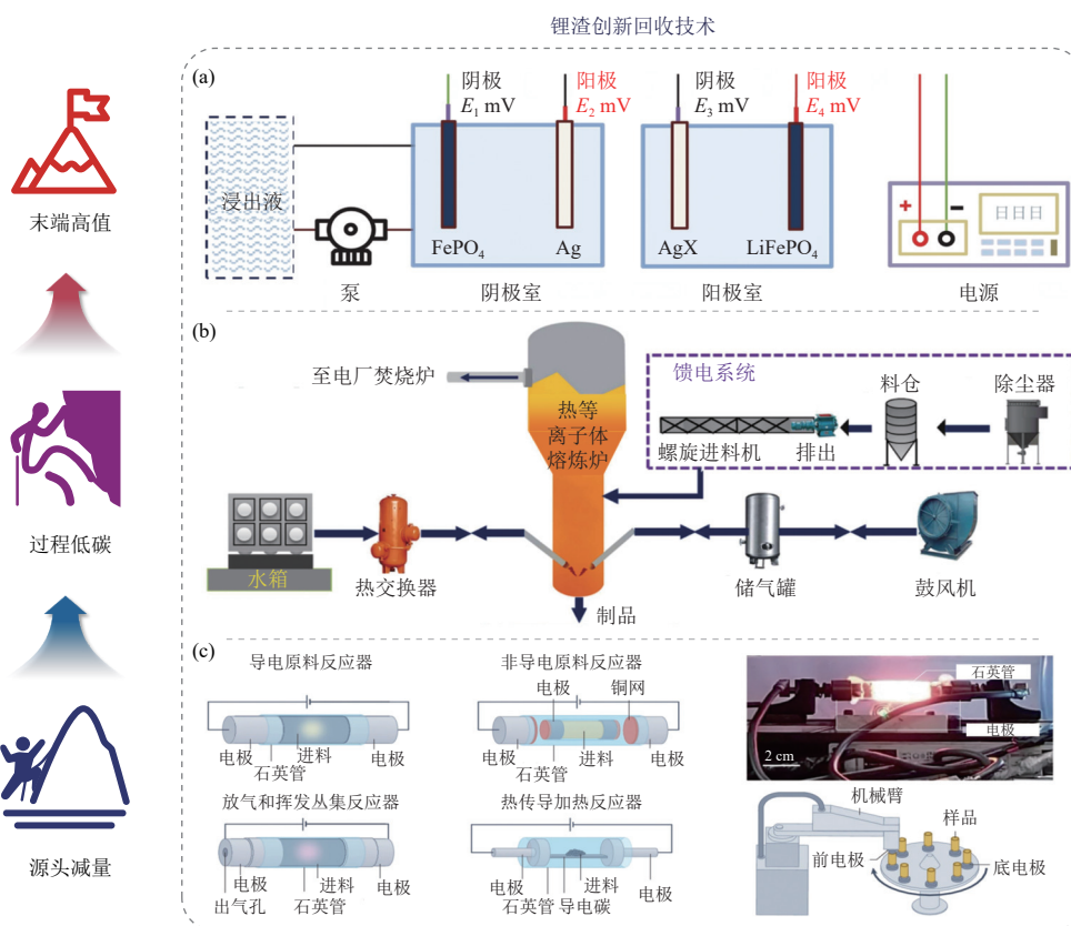
图 5 前沿“绿色”锂矿冶炼渣处理技术 [45-47]
