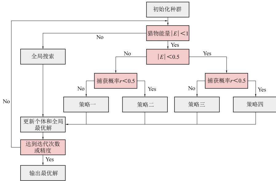
图 1 哈里斯鹰优化算法流程示意图
