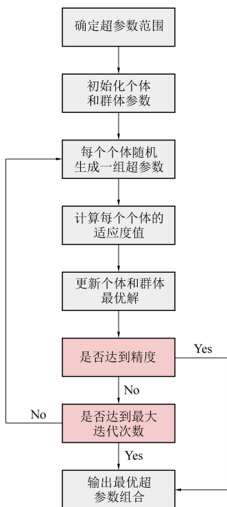
图 3 HHO 优化 CNN-LSTM 模型流程示意图
